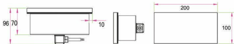
Drawings(mm)
