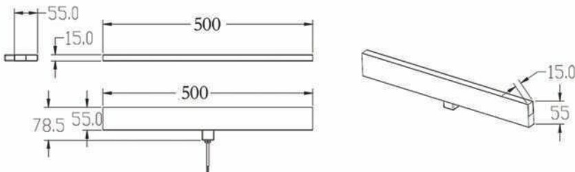
Drawings(mm)
