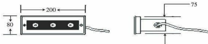
Drawings(mm)
