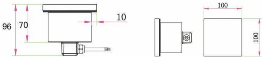
Drawings(mm)
