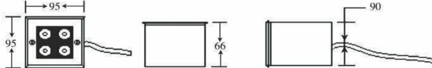
Drawings(mm)
