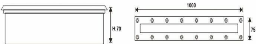
Drawings(mm)
