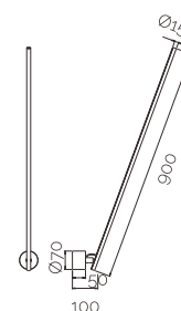
9081 WALL 900
